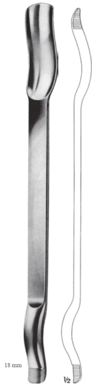
MURPHY-LANE 59-312 Luksasyon elevatörü Luxation lever 33 cm
