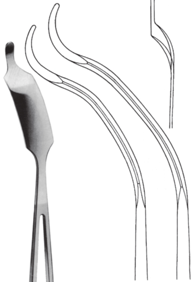
1/2 LANGE-HOHMANN 26.5 cm // 28 cm
